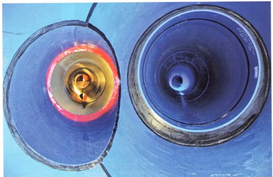
Mit Harz8 abgedichteter Ringspalt.
